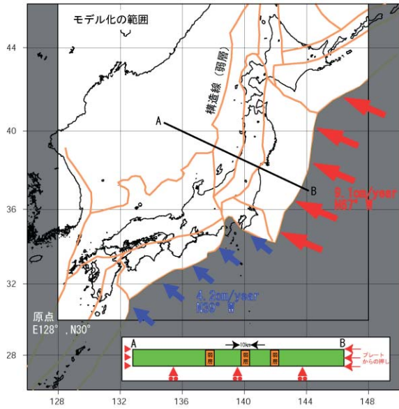
図1 定常的なプレートの沈み込みに伴う地殻変動を検討した領域 (モデル概念)
