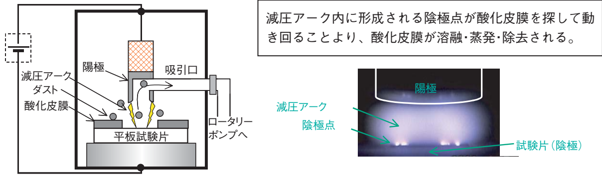
図1 (a) 吸引機構つき減圧アーク除染装置 (b) 減圧アークの様相 (電流60 A、圧力20Pa)
