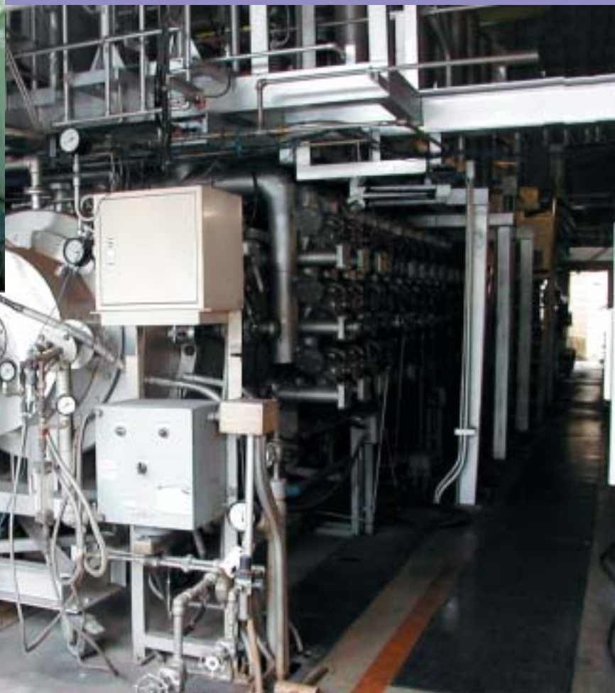
* 石炭燃焼特性実証試験装置 (MARINE炉) (上) と * 石炭燃焼試験設備 (BEACH炉) (下)
